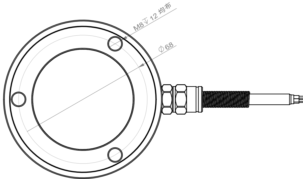
视图 A 比例 1:1
